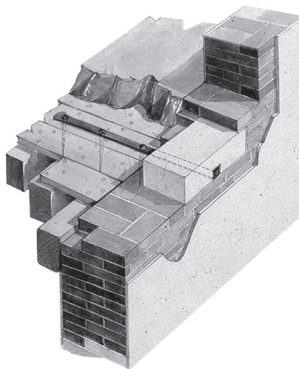
Schema grafico del ruolo dei tiranti, che collegano il solaio al muro esterno e sono un elemento importante nella stabilità degli edifici e ora si stanno ossidando, talora completamente
